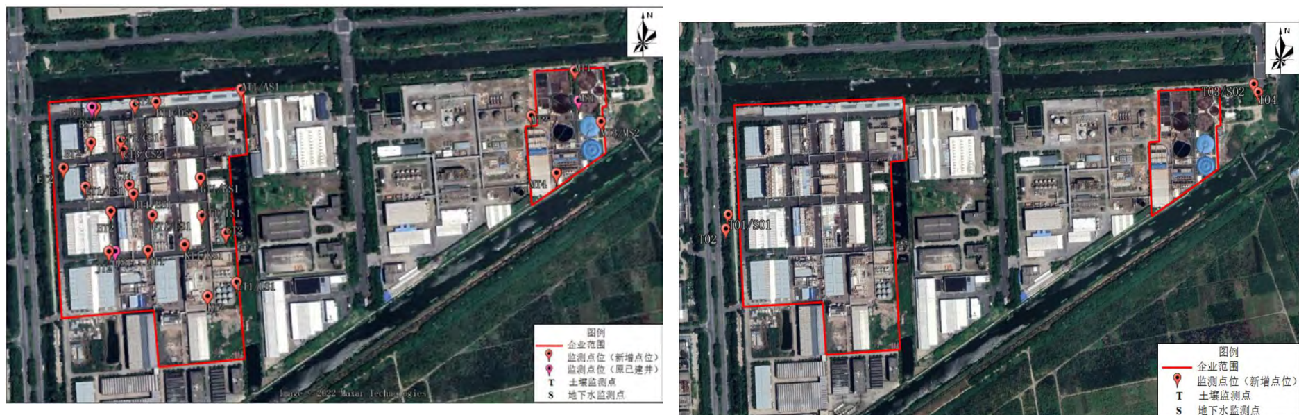
图2.3-2 土壤和地下水监测点位分布图
